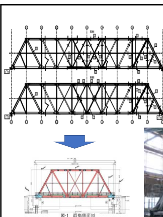
図-1 断面側面図
