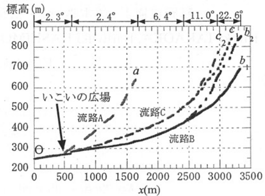
図-5 流路の縦断面図
