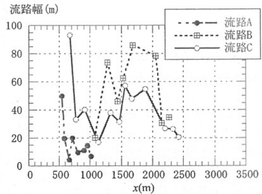
図-6 流路幅の測定値
