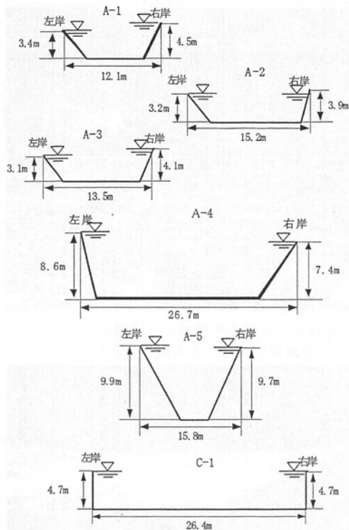
図-8 災害後の流路横断面
