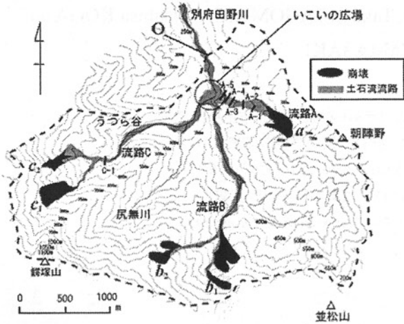
図-4 鰐塚山周辺の平面図
