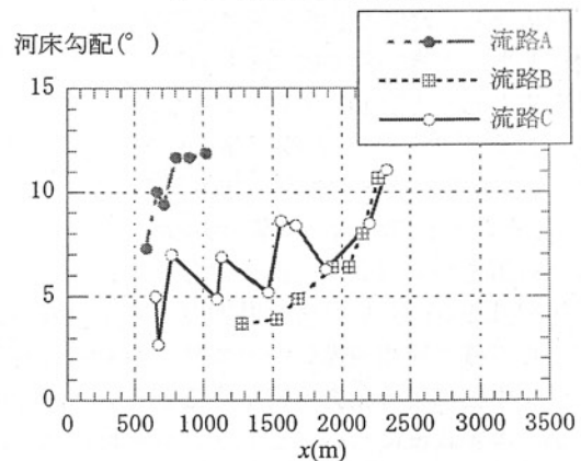
図-7 土石流通過後の河床勾配
