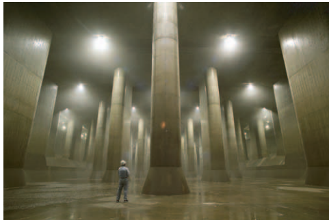
首都圏外郭放水路 (撮影：西澤丞氏)
