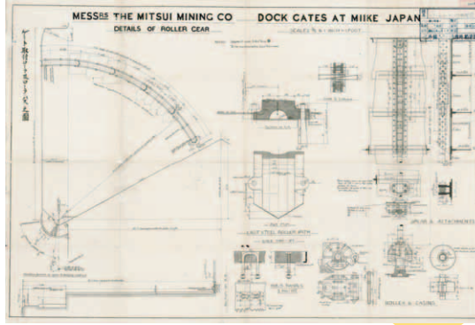
三池港 ゲート部図面
