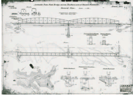
南河内橋 全体平面図
