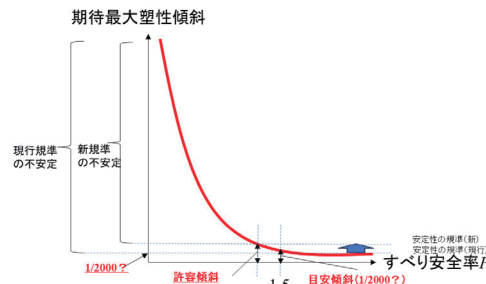
図1 すべり安全率と変形（期待値）の関係
