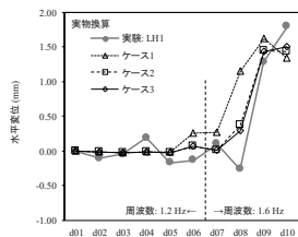
図2 動的的非線形解析による建屋の水平変位の評価
