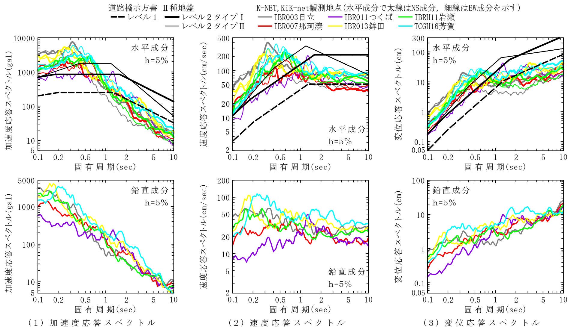
図 ー 2011.03.11 14:47 東北地方太平洋沖地震(M9.0, 深さ24km)の応答スペクトル
