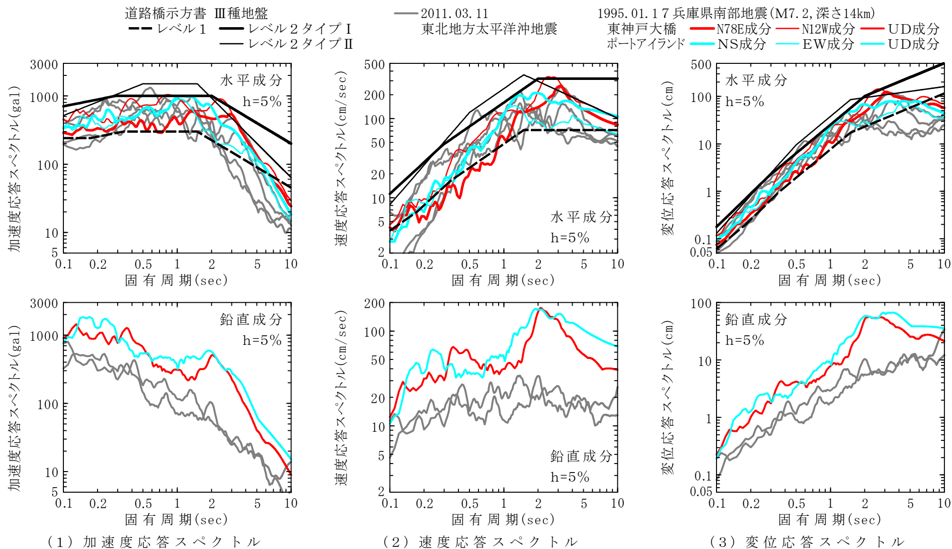
図 — 2011.03.11 14:47 東北地方太平洋沖地震 (M9.0, 深さ24km) の応答スペクトル
