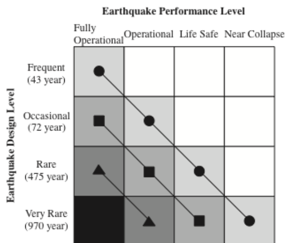
図-5 Vision 2000によるパフォーマンスマトリクス
