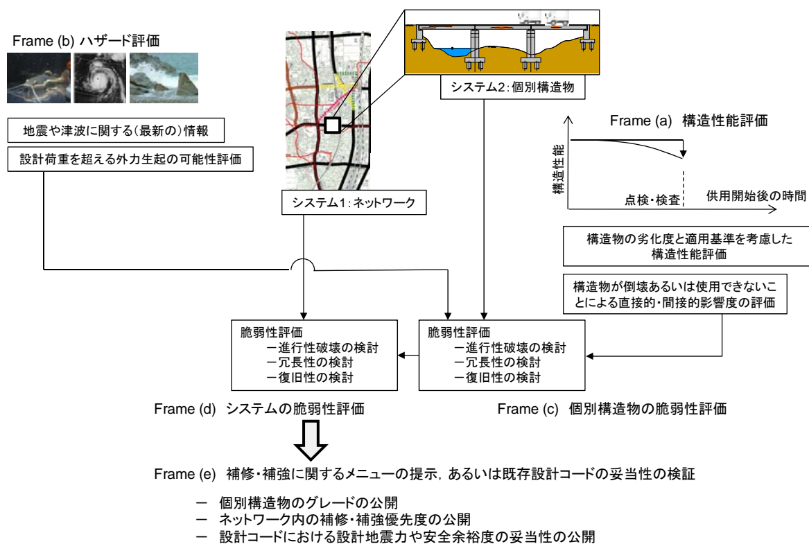
図-8 構造物を含むネットワークの脆弱性評価の流れ
