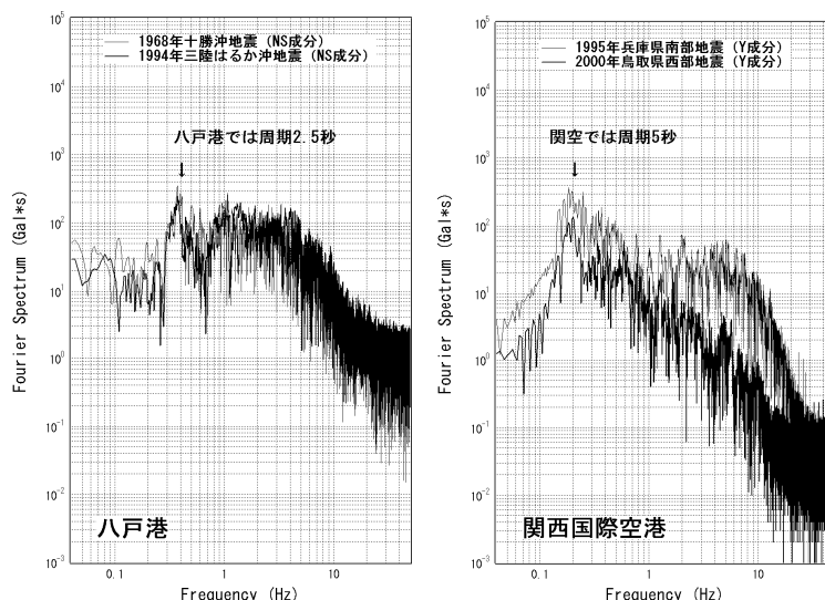
図-4 八戸港と関西国際空港で観測された強震記録のフーリエスペクトルの比較 8)
