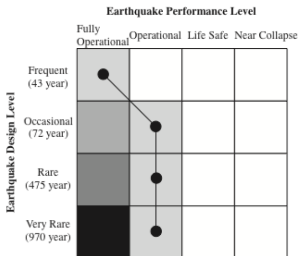
図-6 家村による公共構造物の要求耐震性能案 (担当：高橋良和)
