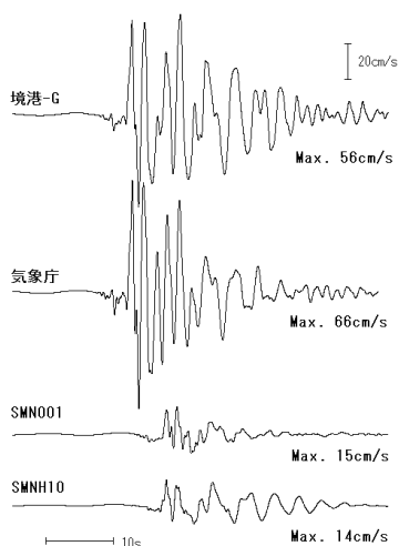
図-3 2000 年鳥取県西部地震の際に境港周辺で観測された速度波形（断層直交成分）
