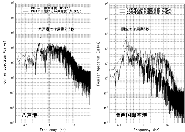
図4 八戸港と関西国際空港で観測された強震記録のフーリエスペクトルの比較 8)
